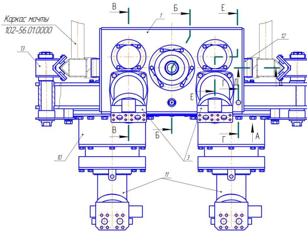
1 – тұрқы (корпус); 2 – сүмбі (шпиндель); 3 – гидроцилиндр; 10 – беру редукторы; 11 – гидромоторлар; 12 – тістегершіктер; 13 – аунақша; 1.1 Сурет – Айналмалы-беру механизмі.
