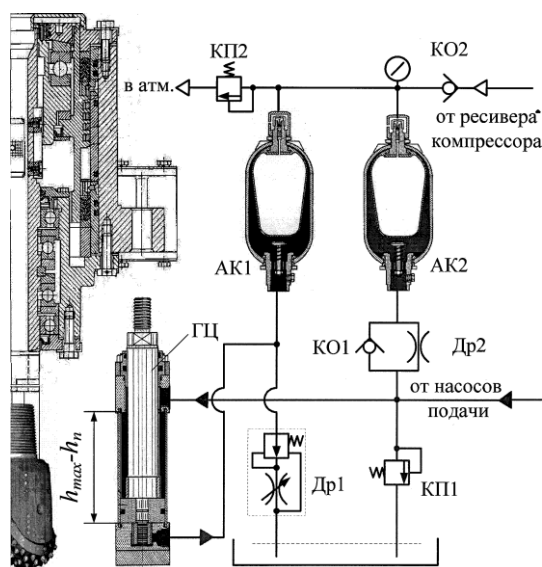
1.4 Сурет – «Бұрғылау станогының айналмалы-беру механизмін берудің инновациялық жүйесінің принципті гидравликалық схемасы»
